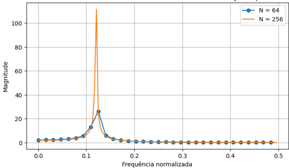
Questão 8 - Influência do número de amostras na resolução espectral
