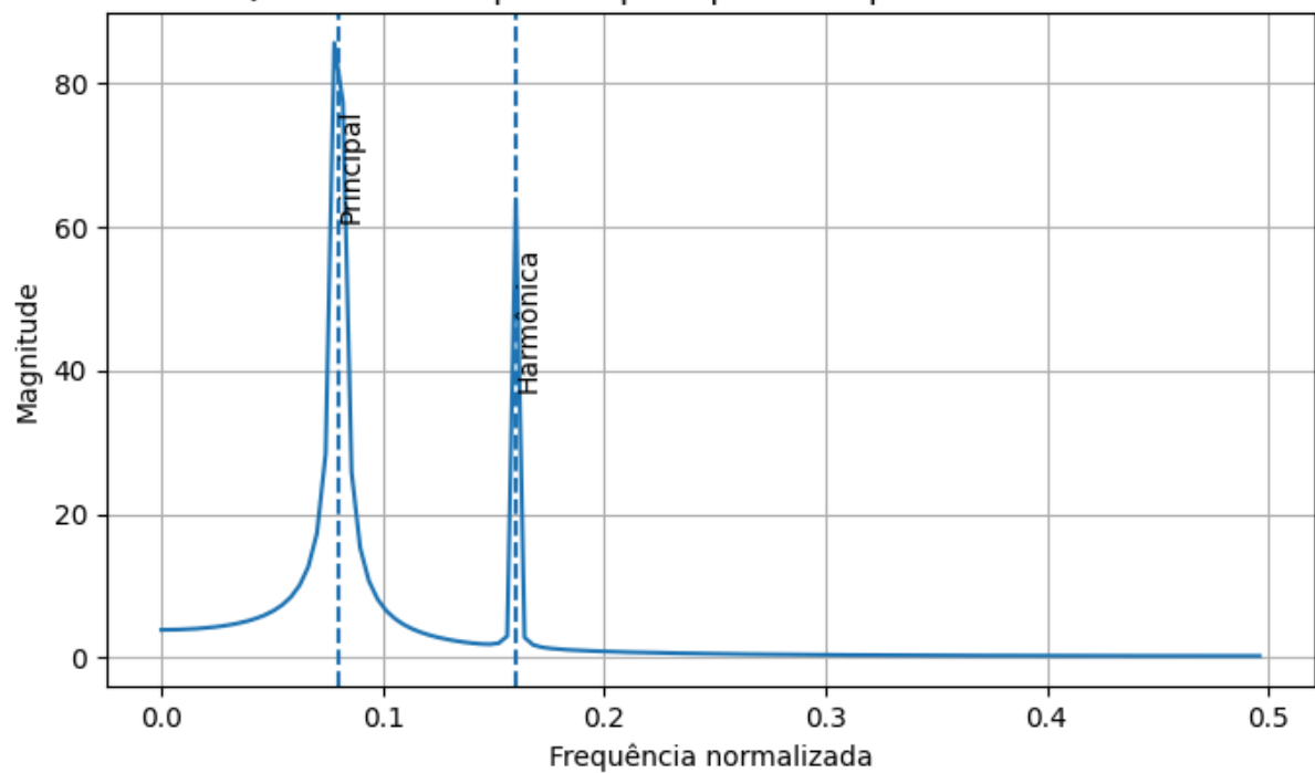
Questão 9 - Frequência principal e componente harmônica
