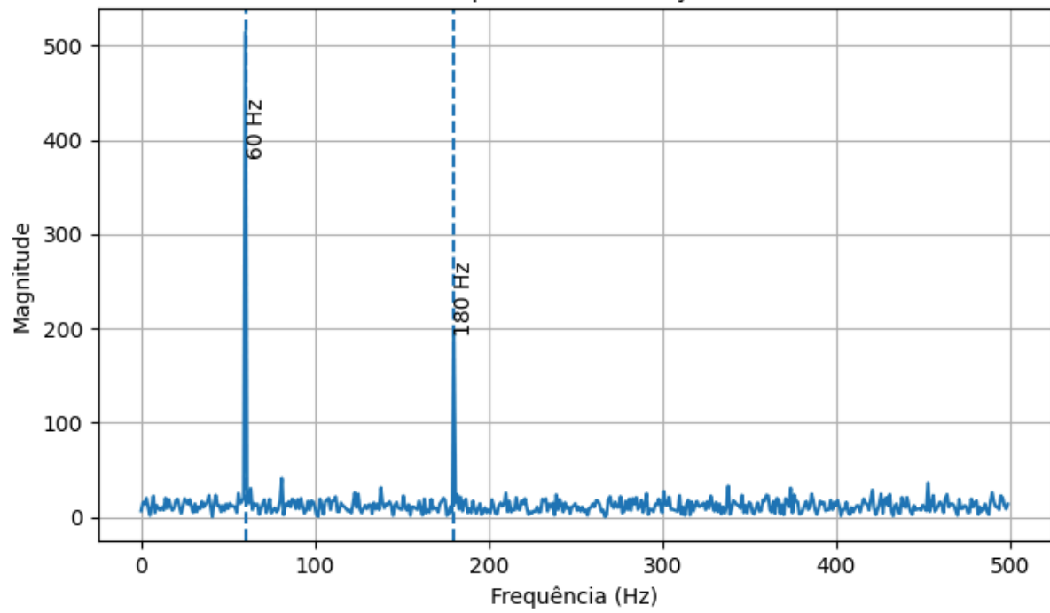
Questão 10 - Análise espectral de vibração simulada com ruído
